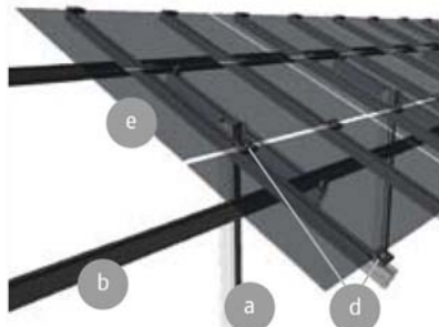
Solar Linea 3 sw σειρών με Φ/Β γεννήτριες χωρίς πλαίσιο
